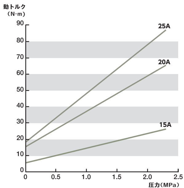
PKシリーズ 動トルク(15A~25A)
