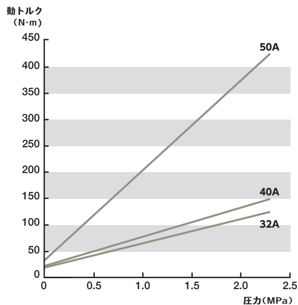
PKシリーズ 動トルク(32A~50A)
