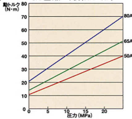
SRK型 動トルク表 (50A~80A)
