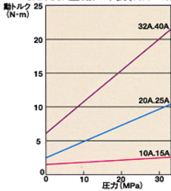
SRK/SSH型 動トルク表 (10A~40A)
